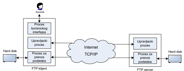
Slika 20 – FTP protokol
